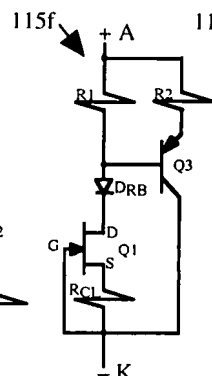
~Prior Art~ FIG. 5F
