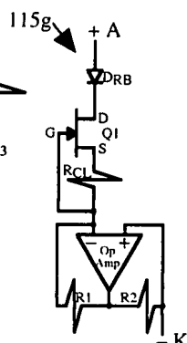
~Prior Art~ FIG. 5G
